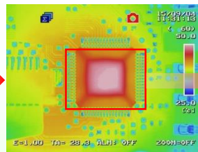
52μm近接拡大レンズ
